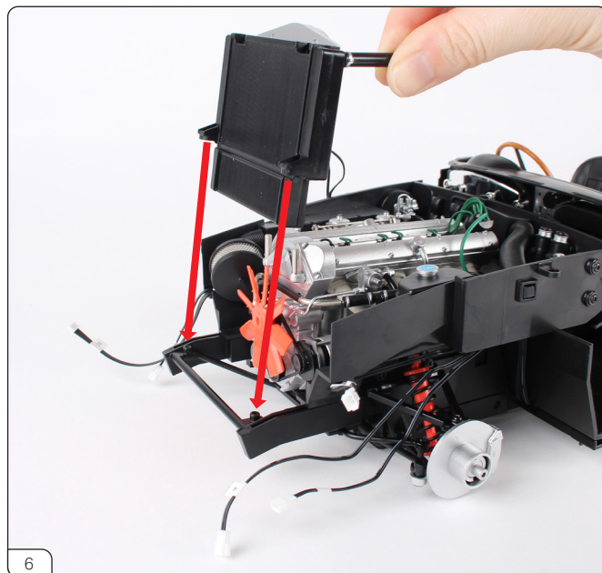
ステージ066で組み立てたシャーシ全面のネジポストに、アッセンブリーを合わせます (赤矢印)。
