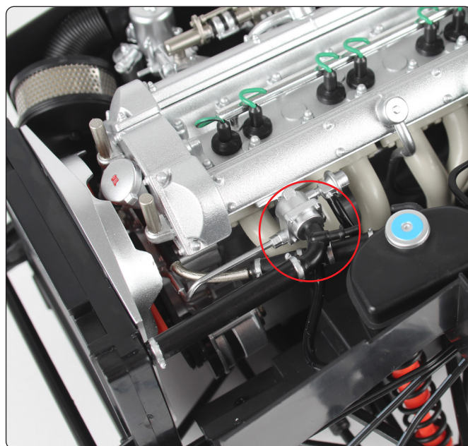
パイプ (96-B) を冷却水サーモスタットにはめ込みます (赤丸印)。
